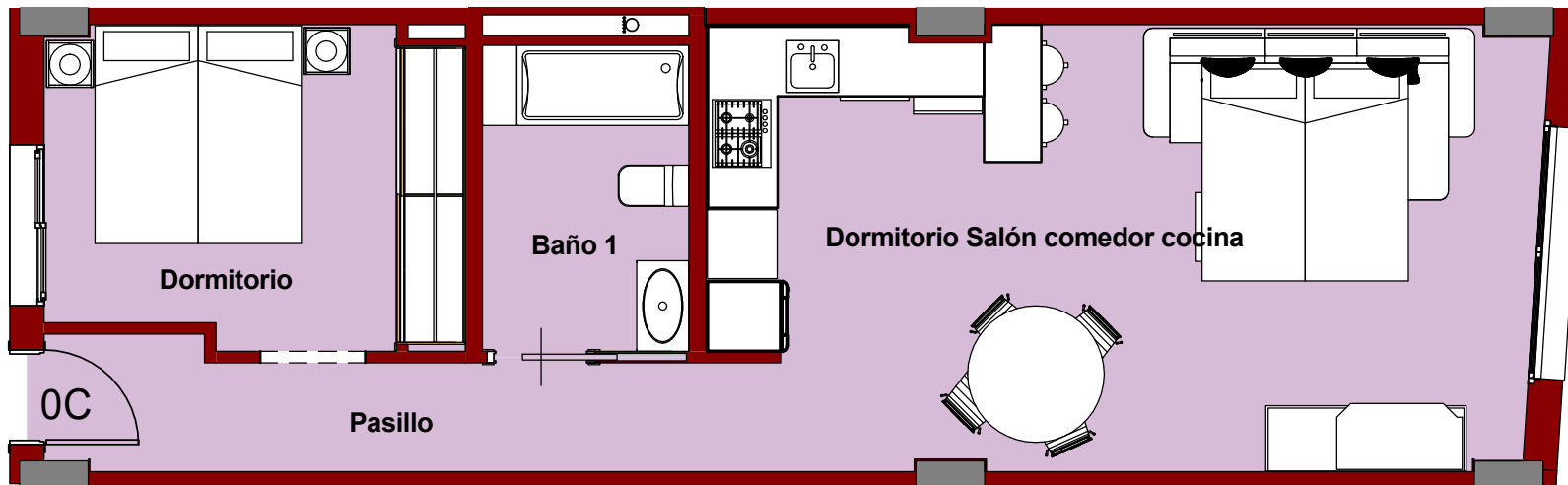
VIVIENDA C - PLANTA BAJA
